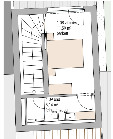
1. OBERGESCHOSS
